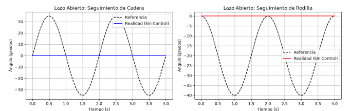
Figura 3. Divergencia de las trayectorias articulares en Lazo Abierto.
