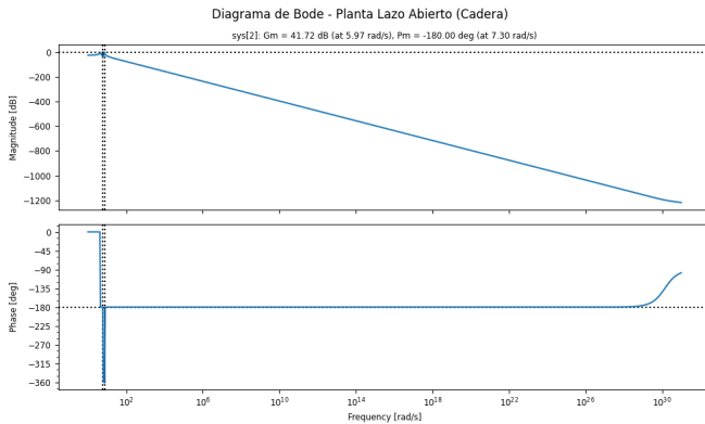
Figura 1. Diagrama de Bode en Lazo Abierto.
