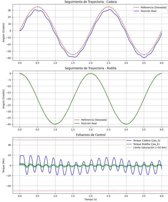
Figura 5. Seguimiento articular y esfuerzo de control - Frecuencia.
