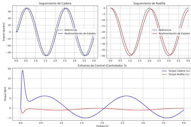
Figura 6. Seguimiento articular y esfuerzo de control - Realimentación de Estados.
