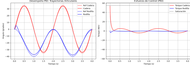
Figura 4. Seguimiento articular y esfuerzo de control - PID.
